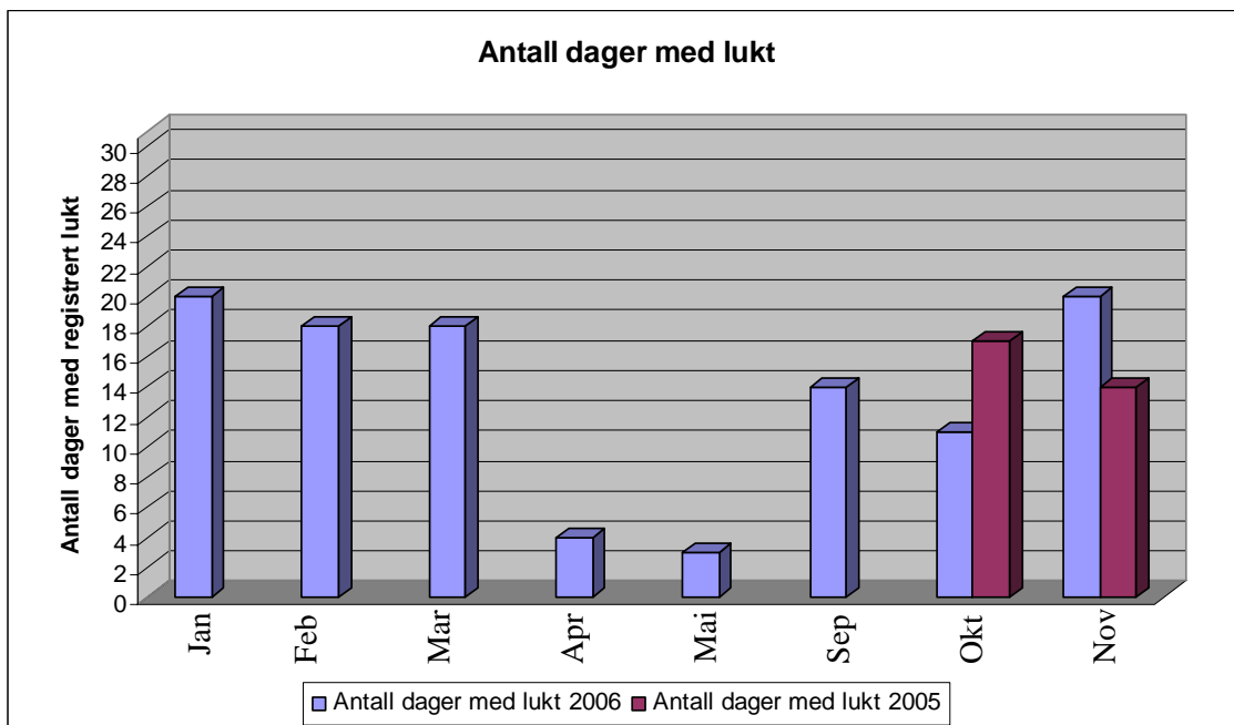
Figur 1: Presentasjon av antall dager pr måned hvor lukt er registrert av en eller flere deltakere i luktpanelet. De blå søylene viser registreringer gjort i 2006, de røde søylene viser registreringer gjort i 2005. Datagrunnlaget er ikke stort, resultatene bør derfor brukes med forsiktighet.
